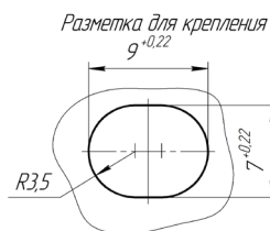
Клемма КП 16
