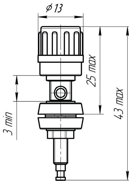
Зажим ЗМП
