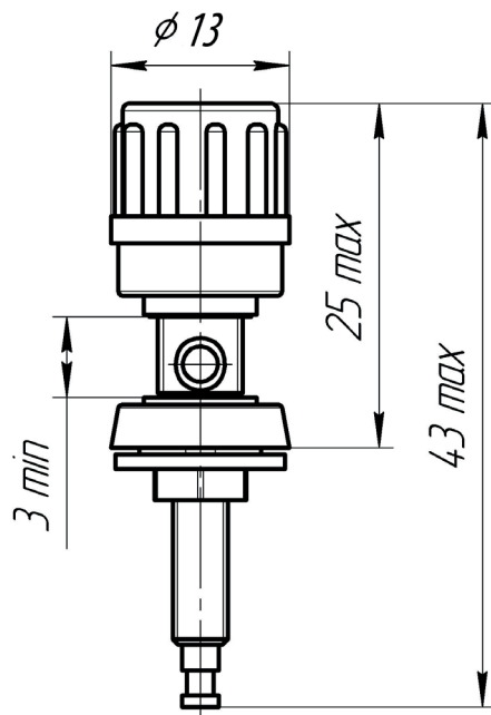
Зажим ЗМЗ
