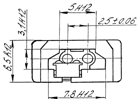
Вилка ОНП-ВГ-3-2/16,3x12 В21
