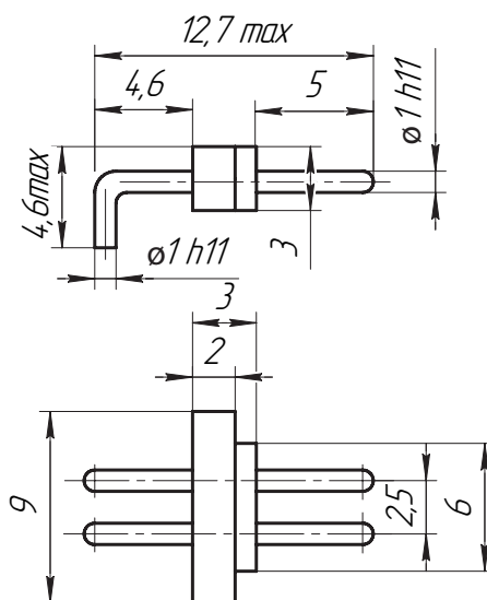
Вилка ОНп-ВГ-2-2/3x9 В21
