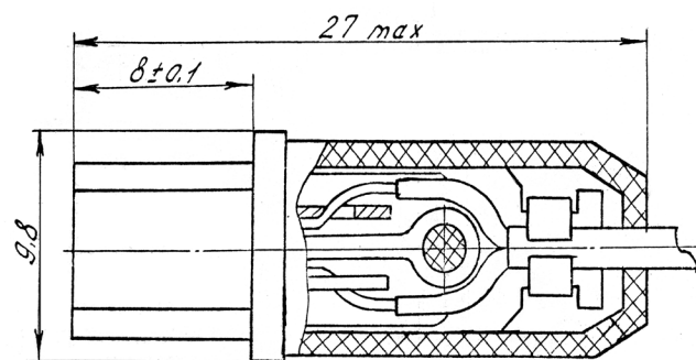
Розетка ОНП-ВГ-2-2/27x9 Р34
